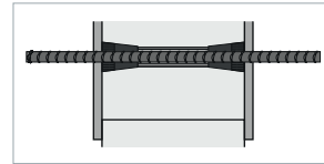
Mod. Tubo rápido encofrado - pasamuro Fast formwork tube Tuyau de passage rapide de coffrage
